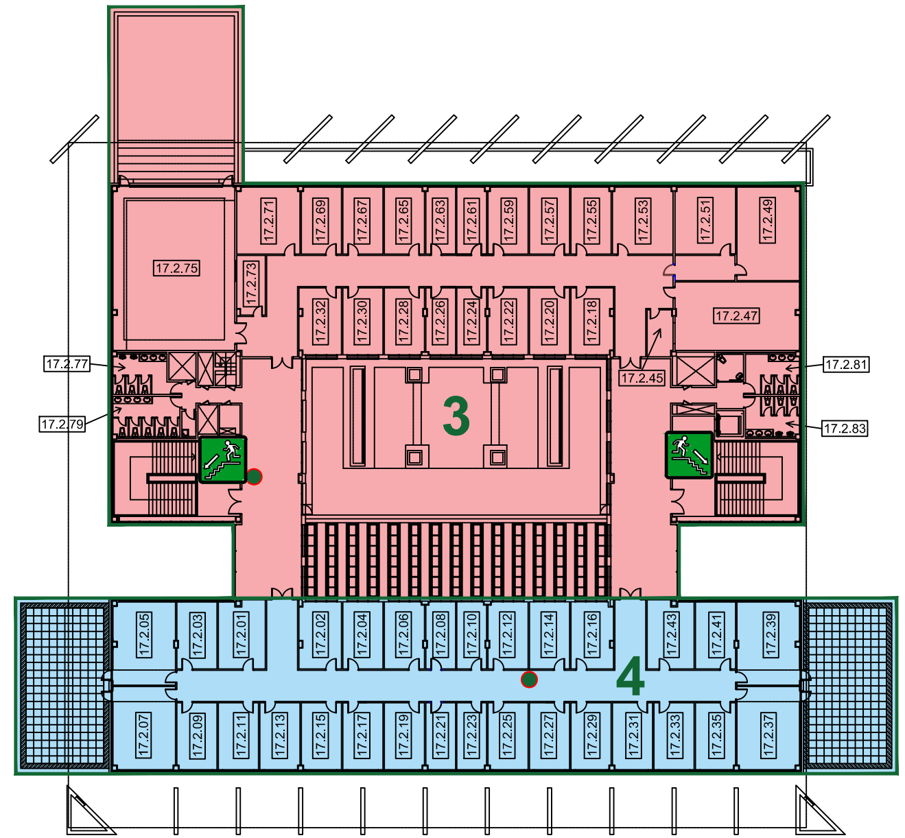
PLANTA SEGUNDA
