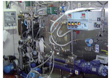
Máquina de absorción; banco de ensayos de componentes para amoniaco
