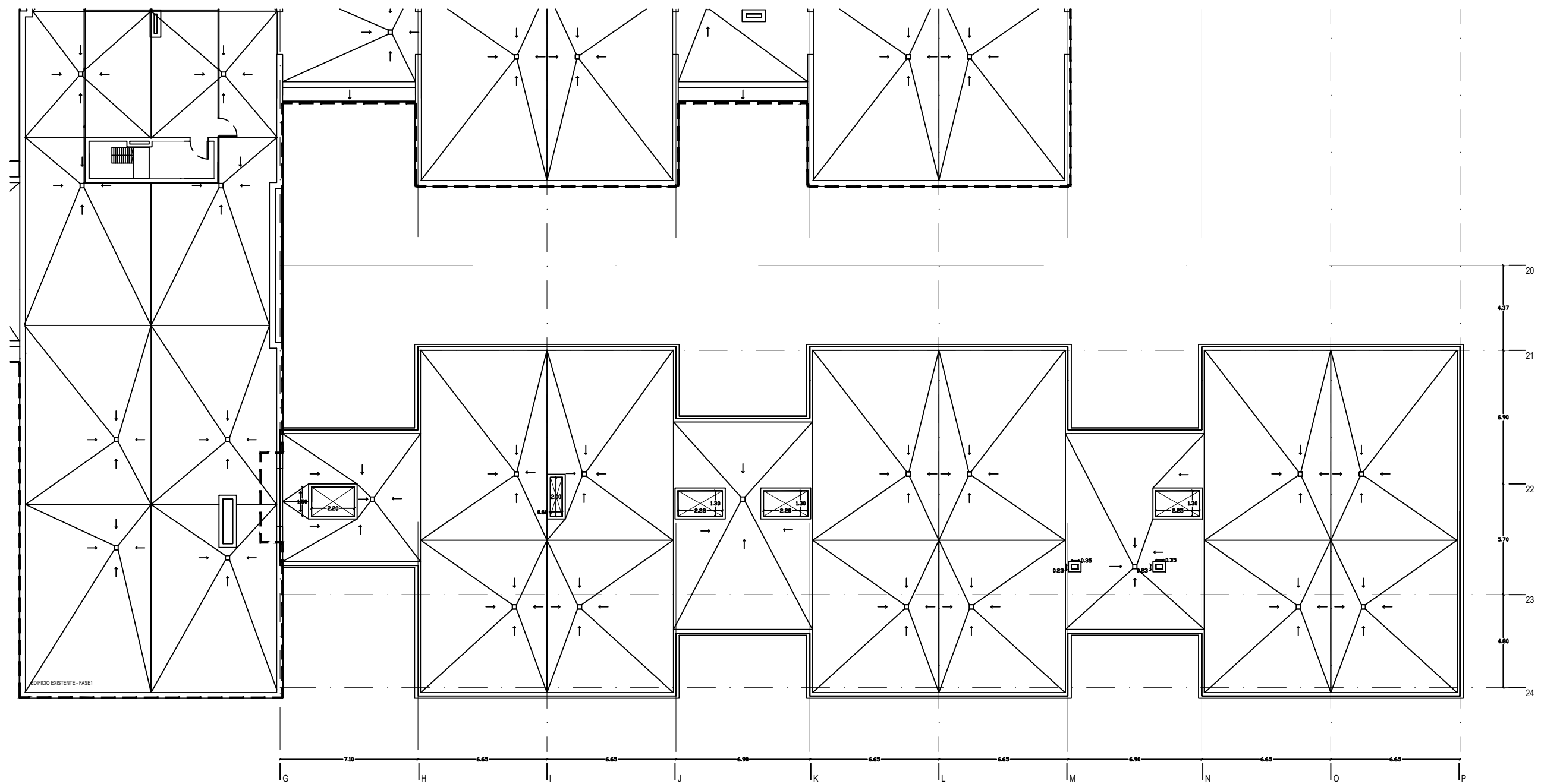
PLANTA NIVEL CUBIERTAS (COTA + 13.30)
