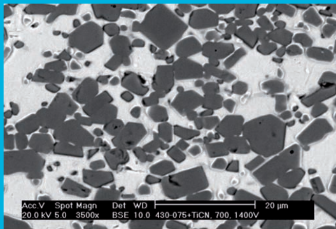
Cermet MATRIX Fe-Cr
