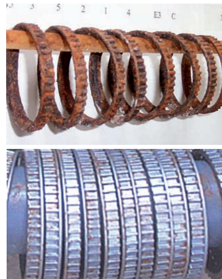
Ensayo de corrosión de anillos ABS de automóvil, fabricados por tecnología de polvos.
