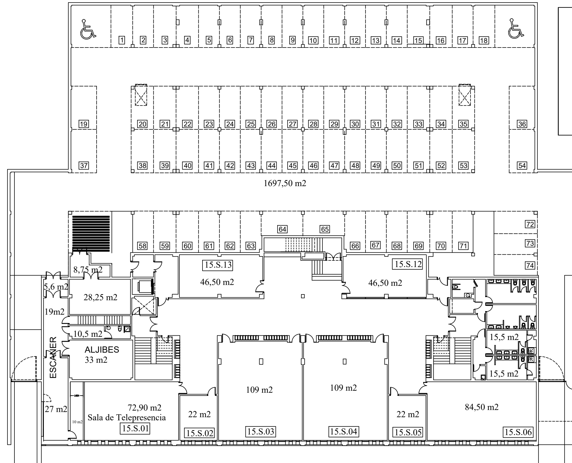
EDIFICIO 15 PLANTA SOTANO
