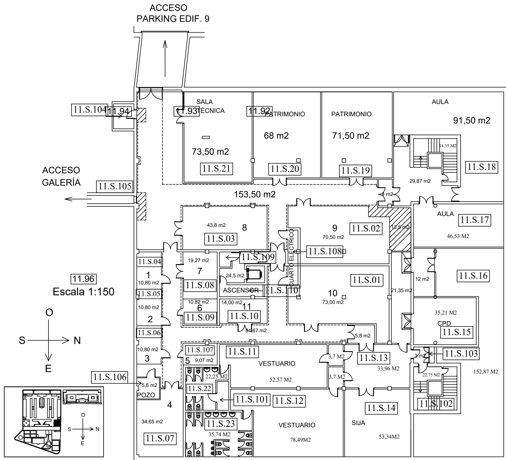
EDIFICIO 11 PLANTA SÓTANO
