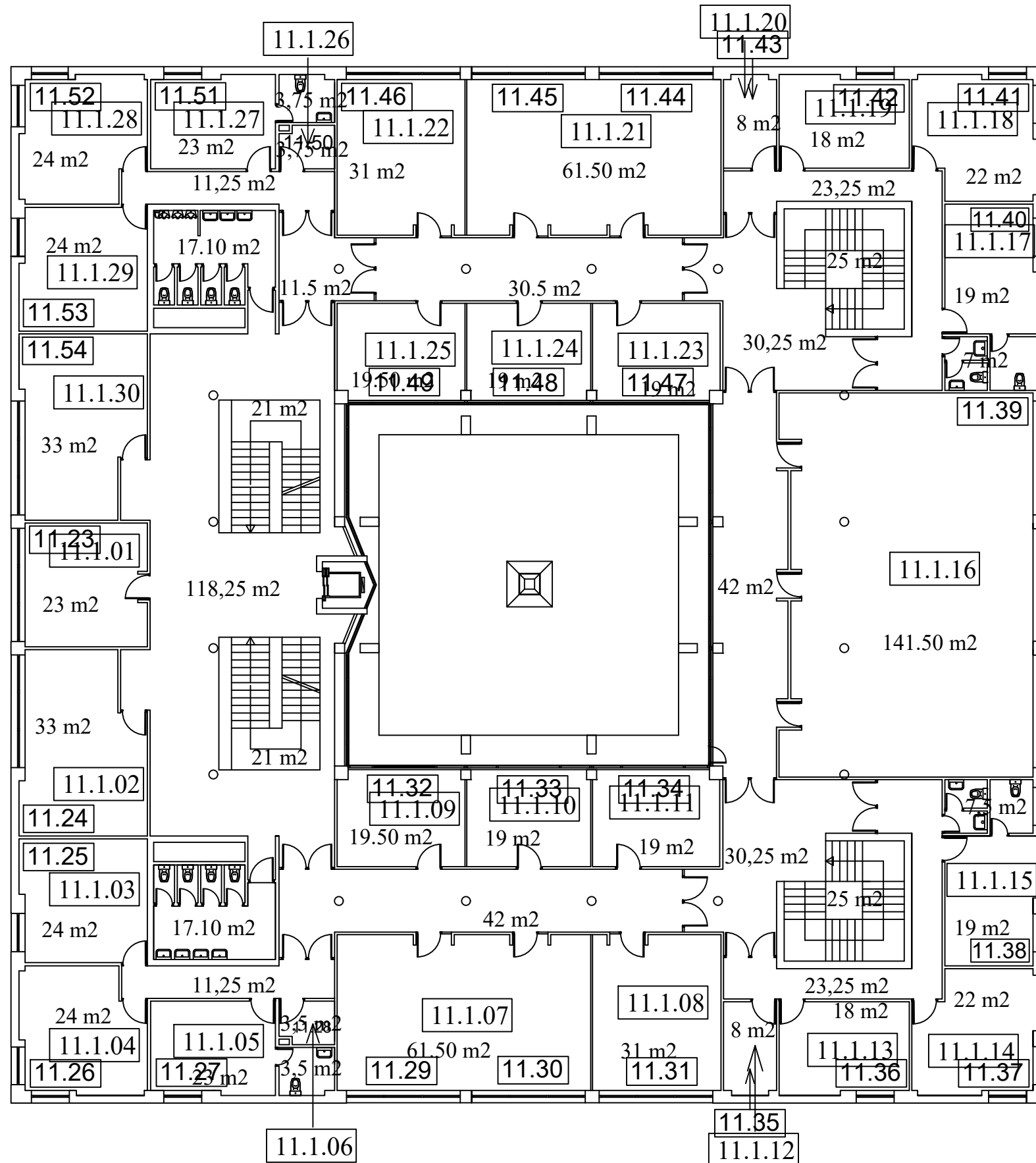
EDIFICIO 11 PLANTA PRIMERA
